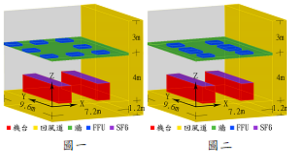
圖一為環型 FFU 無塵室示意圖
