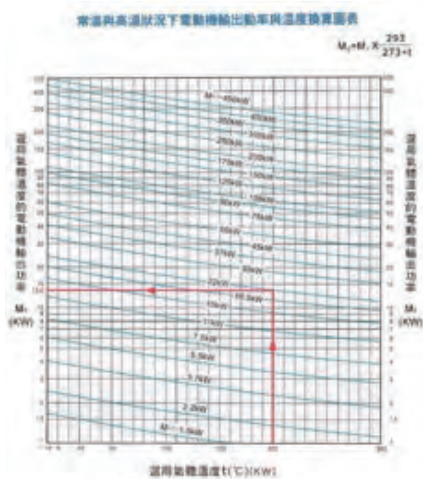
圖2：風車功率隨溫度之變化圖
