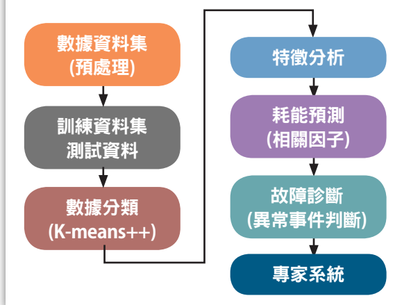
圖4、能源數據AI加值應用分析流程
