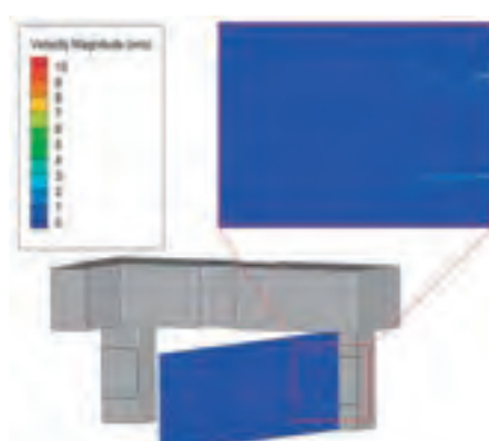
圖4.2風門2mm間隙之洩漏速度分布
