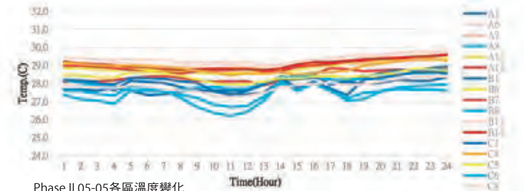
圖八：Phase 2各區溫度分布情況
