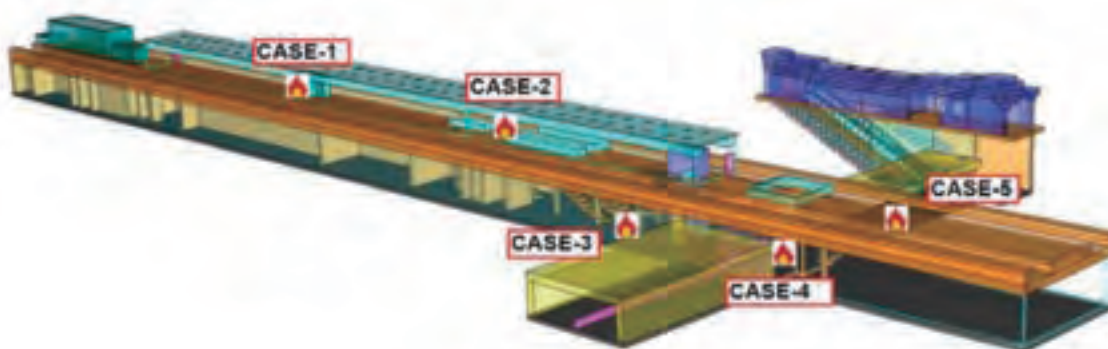
圖3、國外捷運站及捷運車輛火災排煙安全設計模擬
