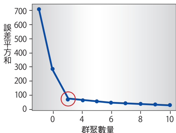
圖6、轉折法分群群數評估圖
