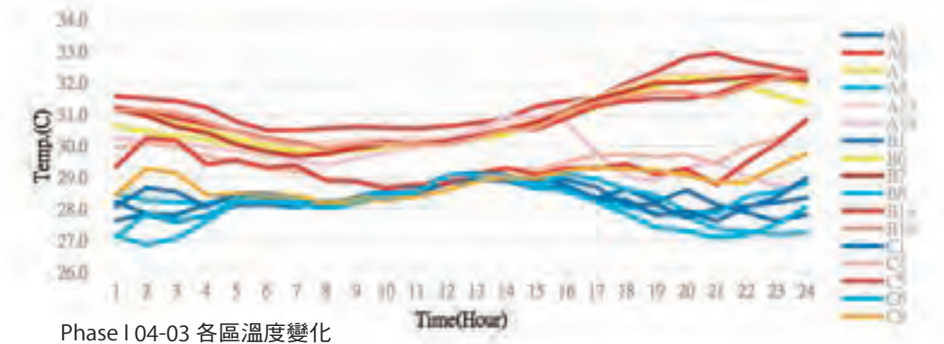
圖七：Phase 1各區溫度分布情況
