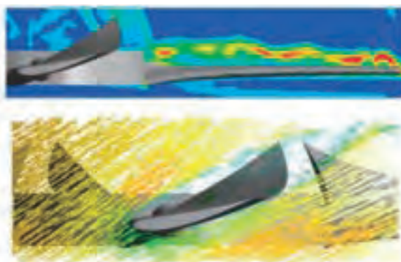
圖2、風扇葉片轉動時的氣流場
