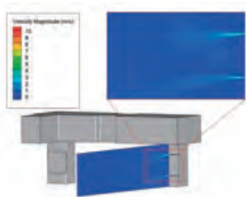
圖4.1 風門5mm間隙之洩漏速度分布
