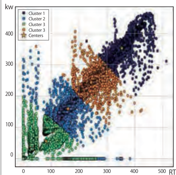
圖11、某工廠冰水主機運轉狀態分類
