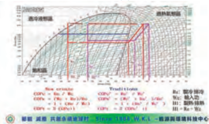
圖7：能量轉換之原理特性圖。
