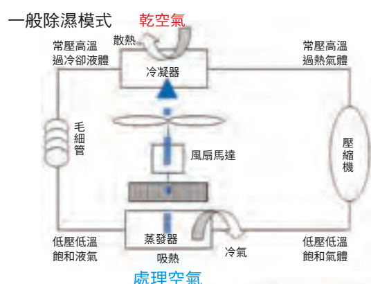
低露點除濕模式
