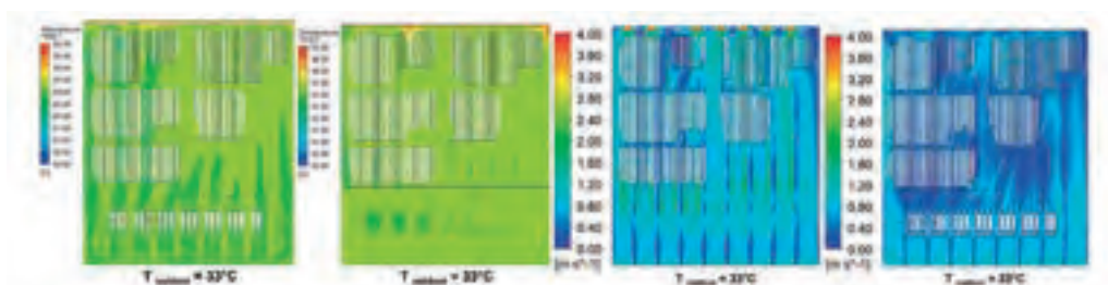
圖五：熱流模擬溫度及速度分布
