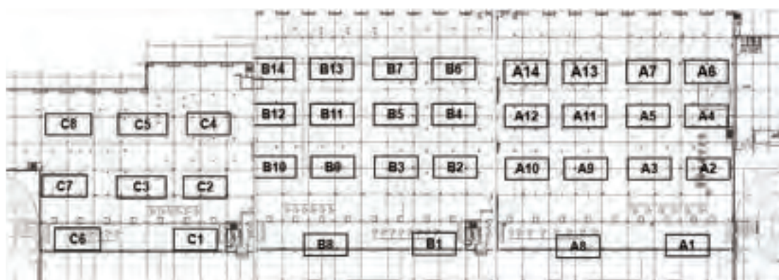
圖二：防火區劃(A/B/C)溫度感測器分布
