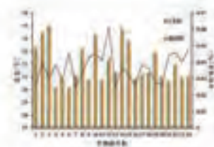
Fluent和ROM的回風口溫度比較圖
