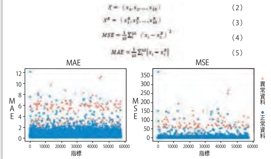
圖9、異常資料檢測還原誤差示意圖
