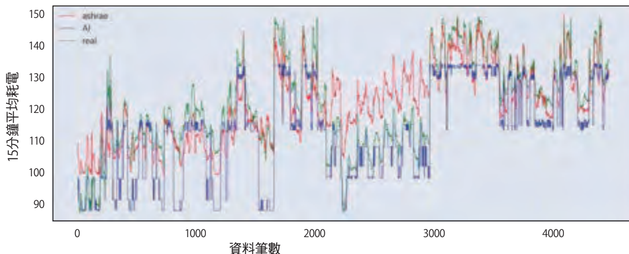
圖13、傳統M&amp;V及AI技術的運轉耗電情形
